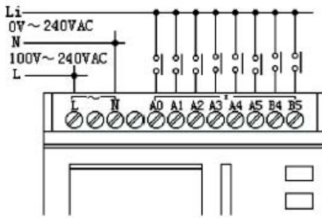
рис. 2.8 тип AC
